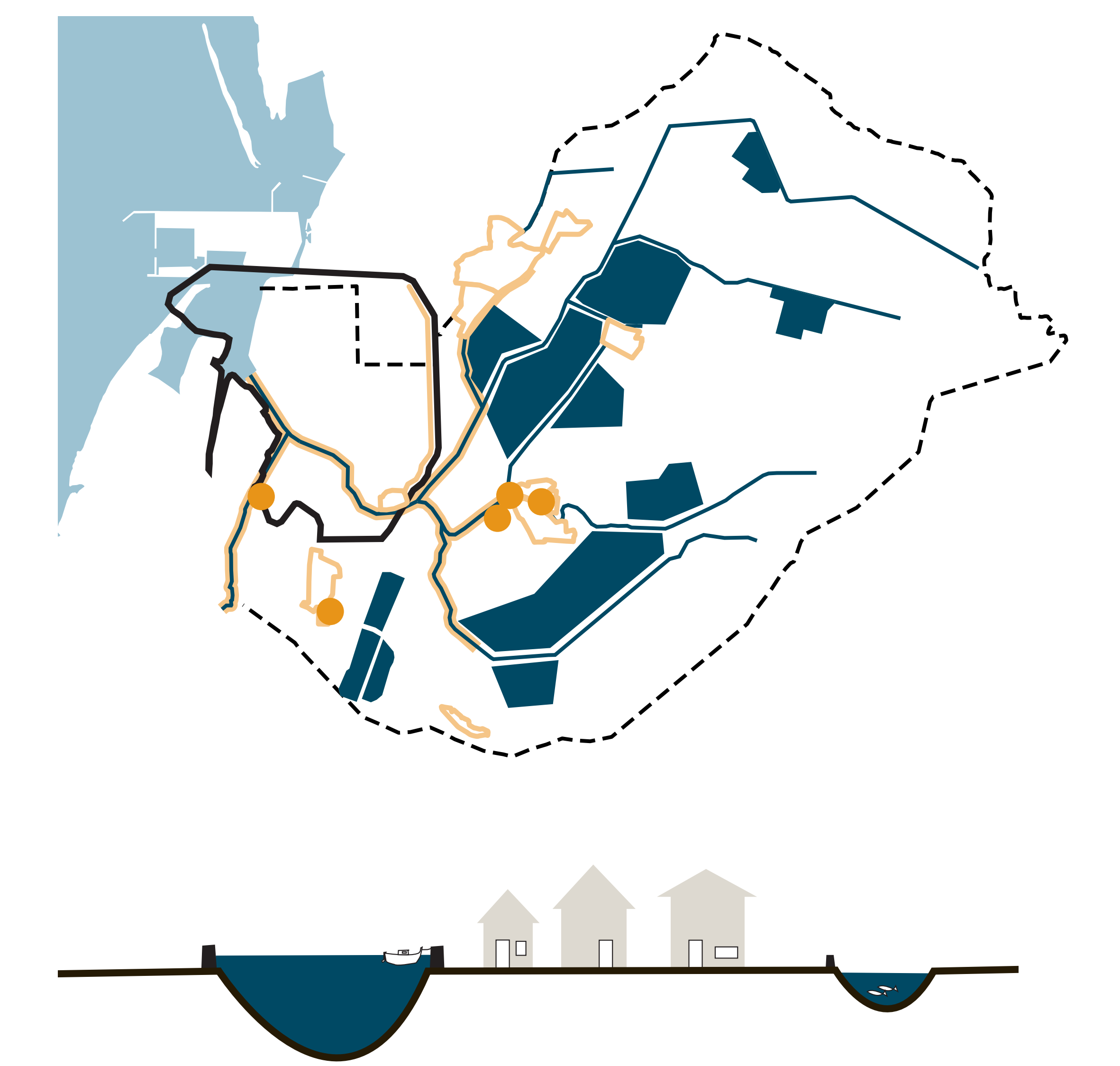
D: upstream detention 上游滯洪池
